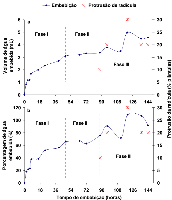
Figura 2. Volume (a) e porcentagem (b) de água embebida e protrusão de radícula (%) durante embebição de sementes de pinhão manso. Petrolina, agosto de 2007.
